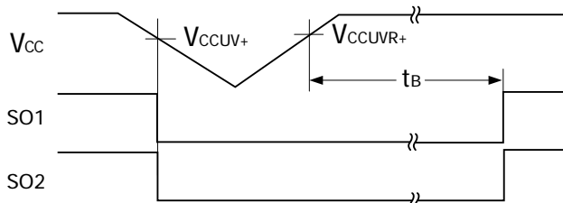
图 7. 原边欠压保护逻辑
