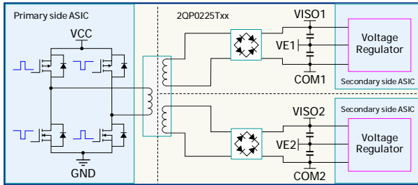
图 6. 供电电路
